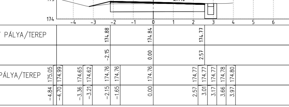
Bán Aladár utca 0+004.00 M=1:100
