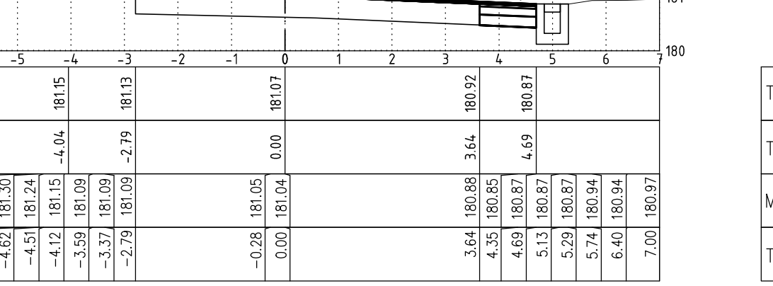
Bán Aladár utca 0+173.00 M=1:100
