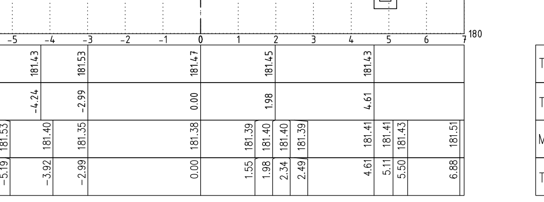
Bán Aladár utca 0+201.00 M=1:100
