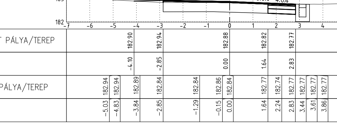
Bán Aladár utca 0+250.00 M=1:100
