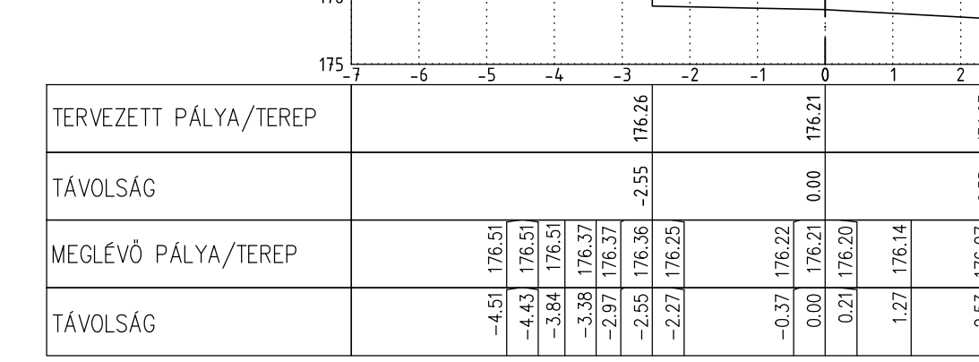
Bán Aladár utca 0+028.00 M=1:100
