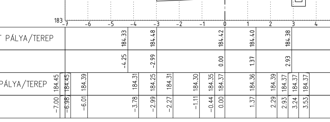
Bán Aladár utca 0+269.73 M=1:100
