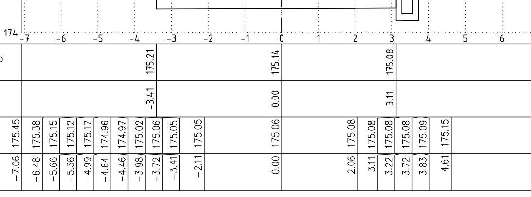
Bán Aladár utca 0+008.15 M=1:100
