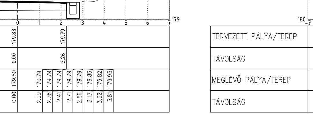
Bán Aladár utca 0+125.00 M=1:100
