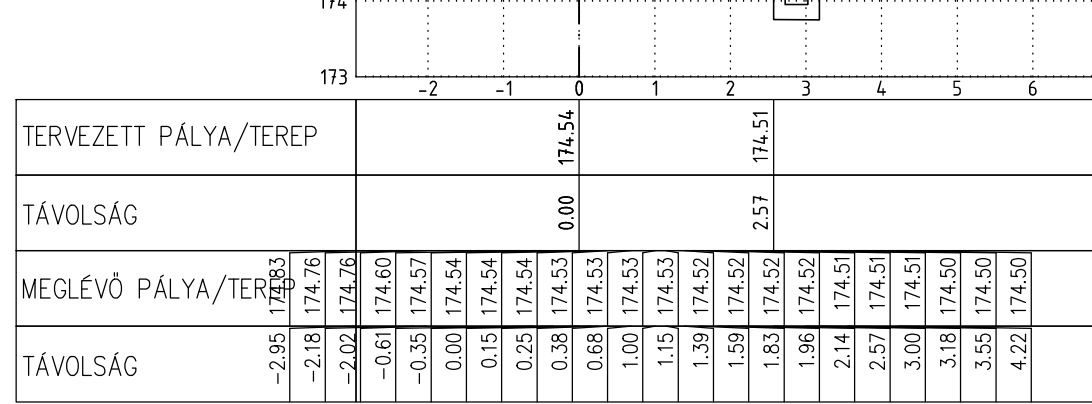
Bán Aladár utca 0+000.00 M=1:100
