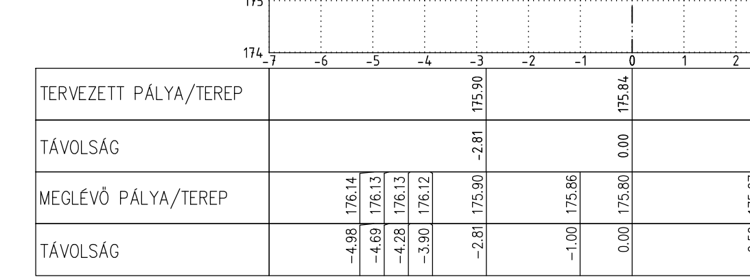
Bán Aladár utca 0+017.73 M=1:100
